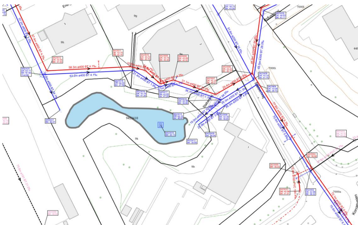
Figur 1: Tegning over regnvandssystem og søen, der anvendes som teknisk anlæg.
